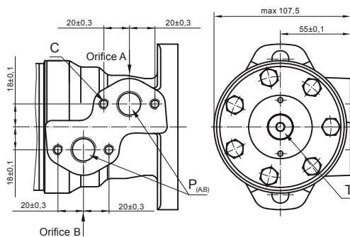
Orifices latéraux
