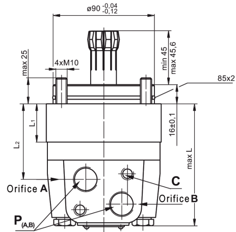
MSV - Montage très court
