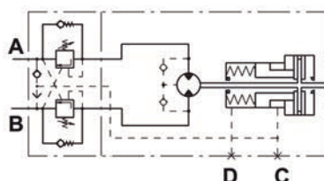
Moteur frein Type TW500B350V
