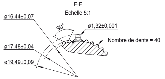
Arbre type "K2"
