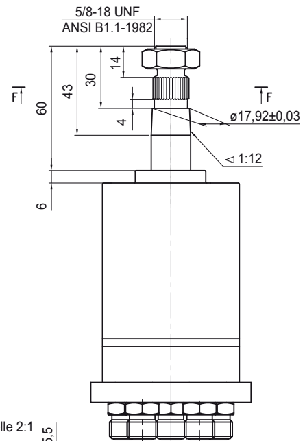
Arbre type "K2"
