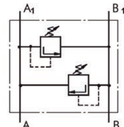
Valve limiteur de pression double, type KPD...
