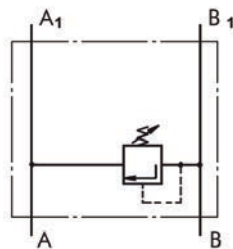
Valve limiteur de pression simple, type KPE...
