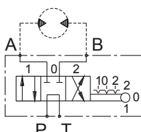
Distributeur 3 positions centre : P vers T - A et B fermés
