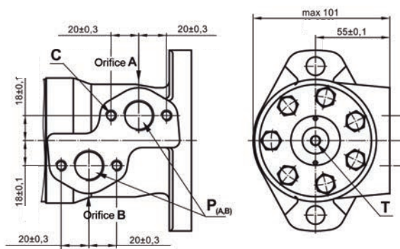
Orifices latéraux
