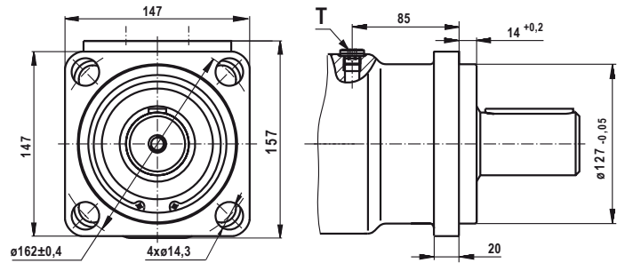
W - Montage roue
