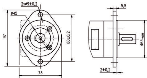
F - Fixation ovale (femelle)
