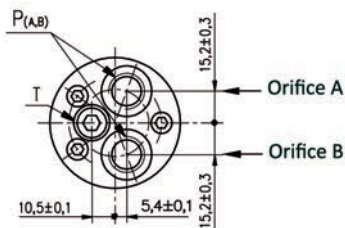
Orifices arrière
