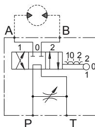
Distributeur 3 positions centre : P vers T - A et B fermés + étrangleur bi-directionnel
