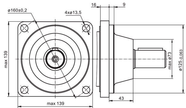
W - Montage roue
