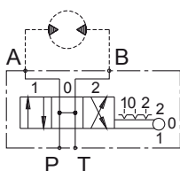
Distributeur 3 positions centre : ouvert
