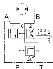
Distributeur 3 positions centre : ouvert + limiteur de pression
