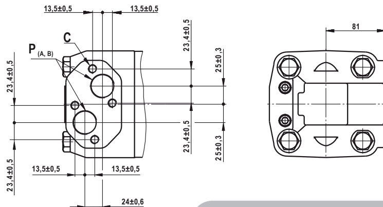
Orifices latéraux
