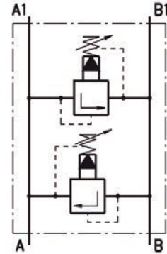
Valve limiteur de pression double, type KPDV...
