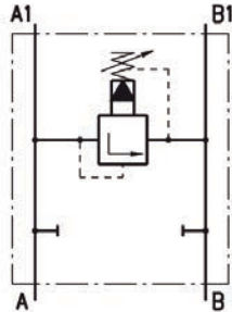
Valve limiteur de pression simple, type KPEAV...
