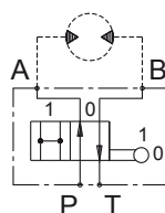
Distributeur 2 positions
