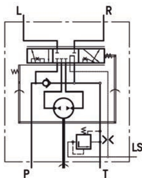
Centre fermé Non réaction de charge HKULR.../5DT
