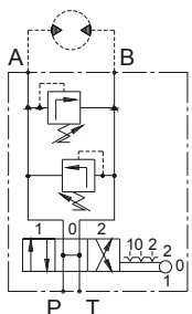
Distributeur 3 positions centre : ouvert + limiteur de pression double
