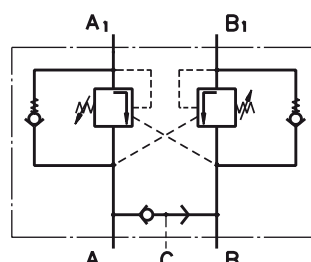
Valve d'équilibrage double avec contrôle de freinage, type KPBR...D
