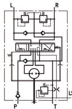
Centre fermé Réaction de charge HKULS.../5DT
