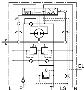
Centre fermé - non réaction Signal statique - HKUS.../SE
