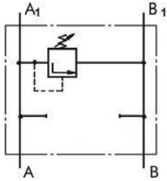
Valve limiteur de pression simple, type KPEAT...
