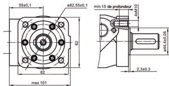
Q - Fixation carrée (4 vis)
