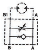
Etrangleur uni-directionnel
