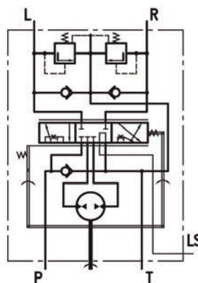
Centre fermé Non réaction de charge HKULV.../5DT
