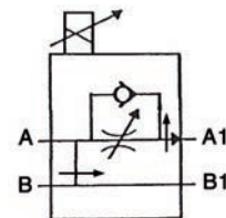
Clapet anti-retour intégré
