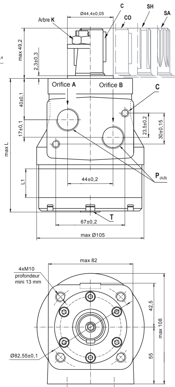
Q- Fixation carrée (4 vis)
