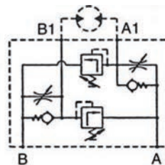
Etrangleur uni-directionnel, double + limiteur de pression double
