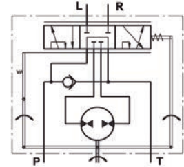
Centre ouvert Non réaction de charge Version 4 - HKU.../4
