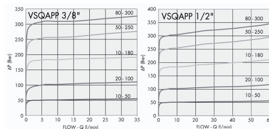
Pression / Débit
