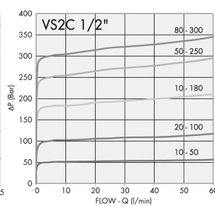
Pression / Débit
