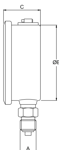
Manomètres raccord vertical
