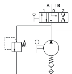
Schéma hydraulique
