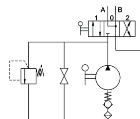
Schéma hydraulique
