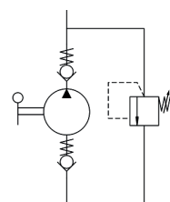
Schéma hydraulique
