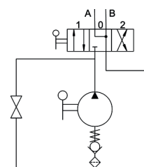
Schéma hydraulique
