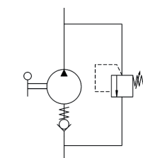
Schéma hydraulique
