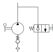
Schéma hydraulique
