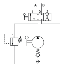
Schéma hydraulique
