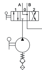
Schéma hydraulique
