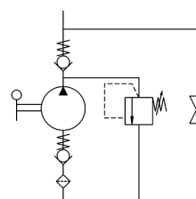
Schéma hydraulique
