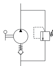
Schéma hydraulique
