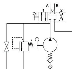
Schéma hydraulique
