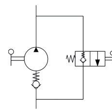
Schéma hydraulique
