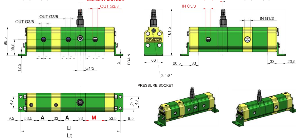
ÉLÉMENTS DU DIVISEUR DE DÉBIT
