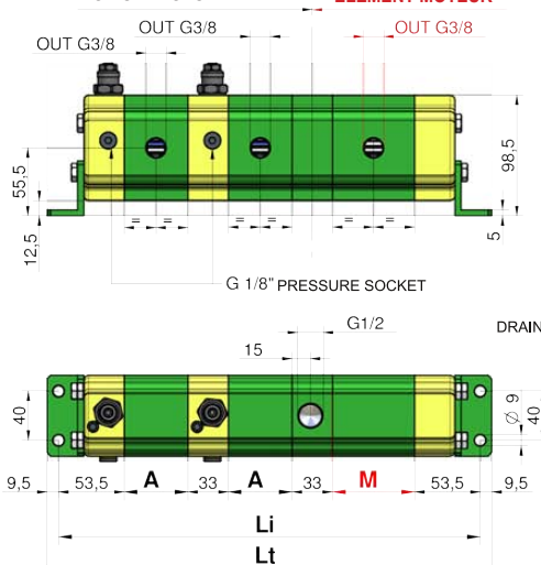
ÉLÉMENTS DU DIVISEUR DE DÉBIT ÉLÉMENT MOTEUR
