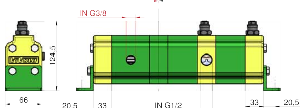
ÉLÉMENT MOTEUR ÉLÉMENTS DU DIVISEUR DE DÉBIT
