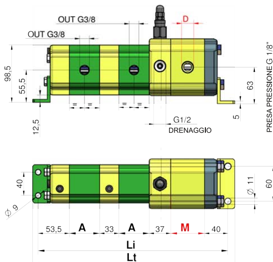
ÉLÉMENTS DU DIVISEUR DE DÉBIT
