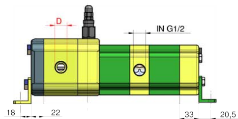
ÉLÉMENT MOTEUR
