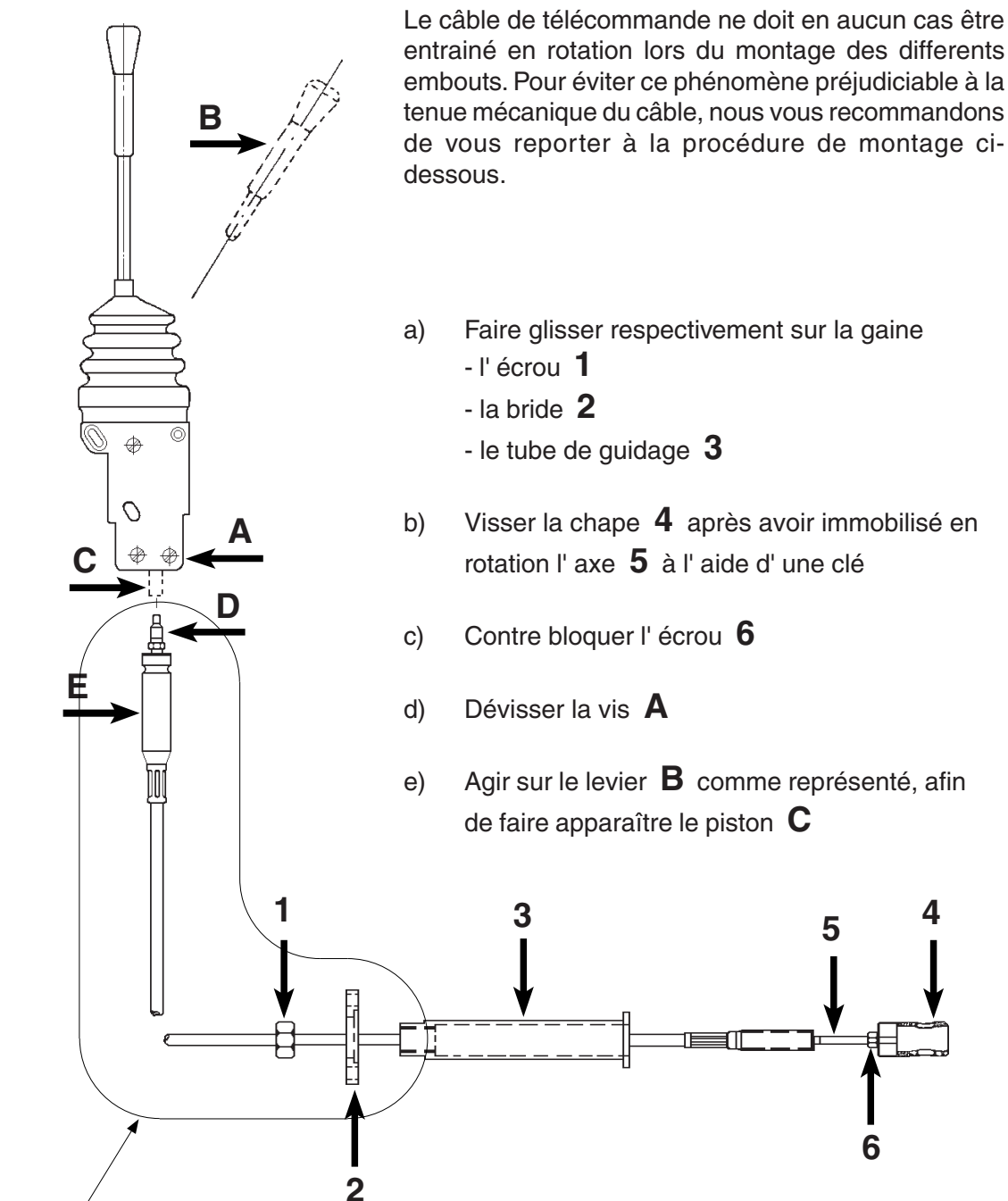
Câbles de commande
