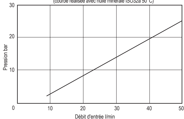
Chute de pression typique (courbe réalisée avec huile minérale ISO32 à 50°C)
