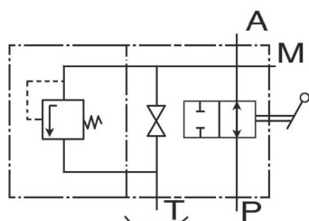
BS 25 - Encombrement décharge manuelle
