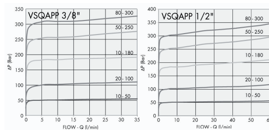
Pression / Débit
