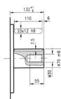
Cylindrique
