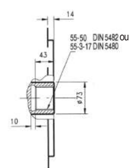
Femelle Cannelé
