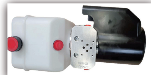
Réf. 141.115.00043 Plaque départ pour flasquer 1 distributeur Cetop 3 sur la minicentrale.
