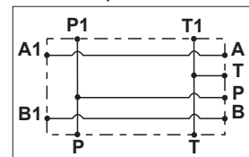
Schéma hydraulique en parallèle
