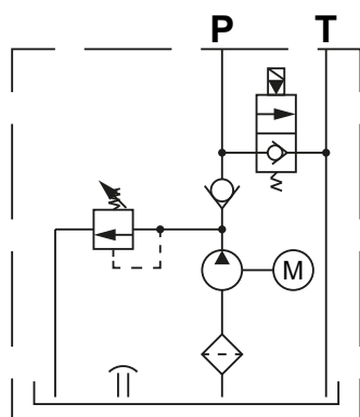
Version avec électrovalve
